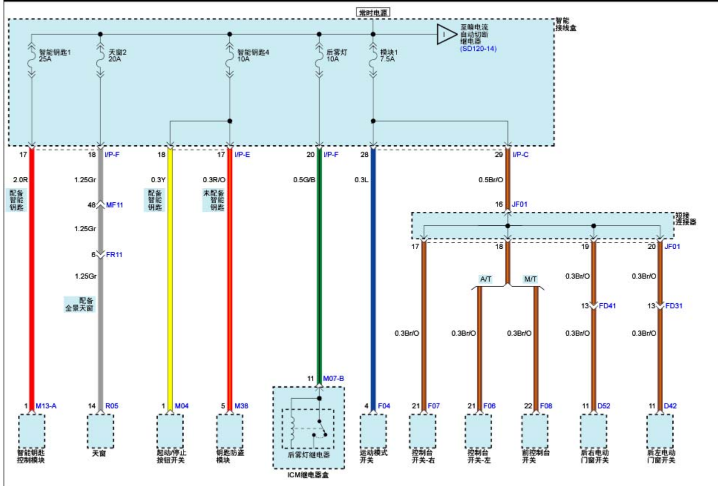
室内保险丝分布(13)
